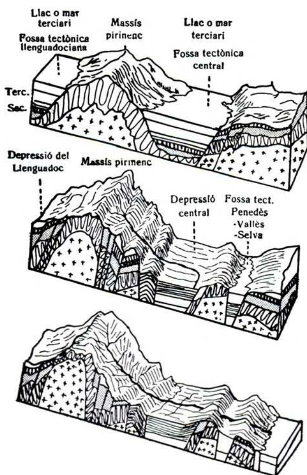
Fig. 2. - Esquema de l'evolució geològica de Catalunya en els temps terciaris i quaternaris.
