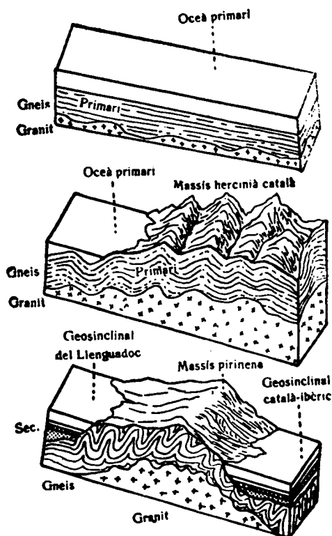
Fig. 1. - Esquema de l'evolució geològica del Pirineu en els temps primaris i secundaris.
