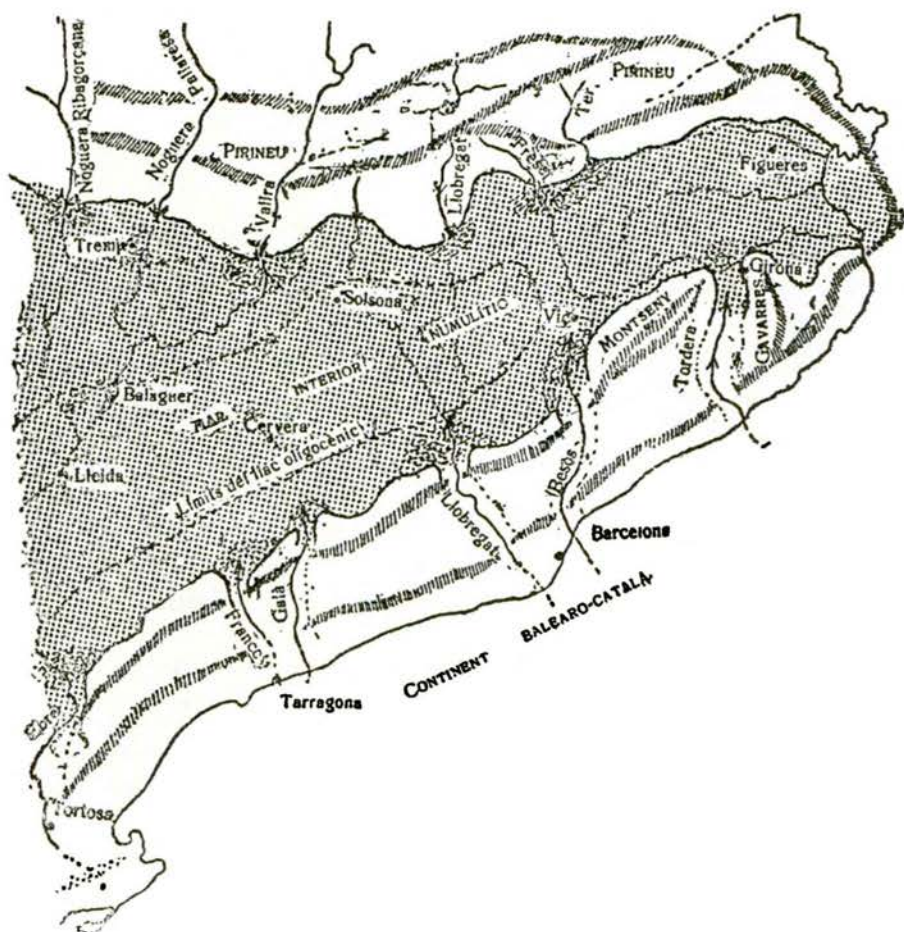
Fig. 7. - Catalunya durant el període numulític, segons Marcel Chevalier.
