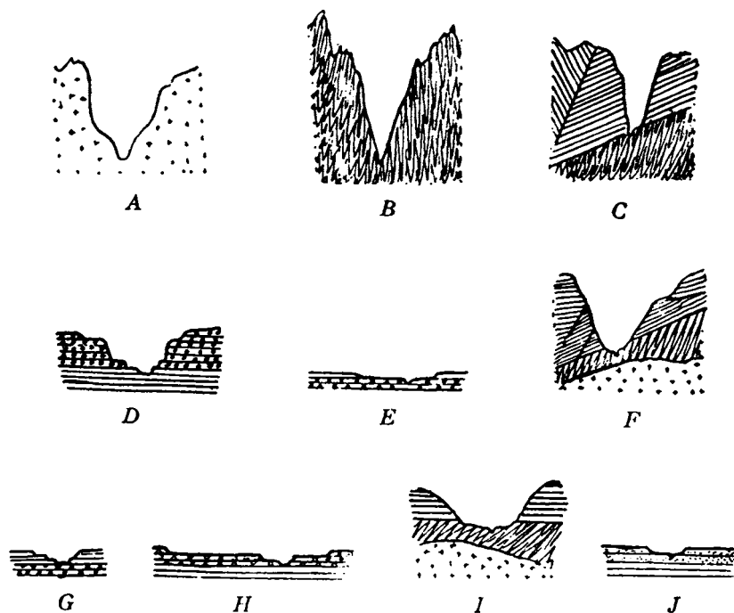
Fig. 8. - Formes de les valls al llarg del curs d'un riu pirinenc,
