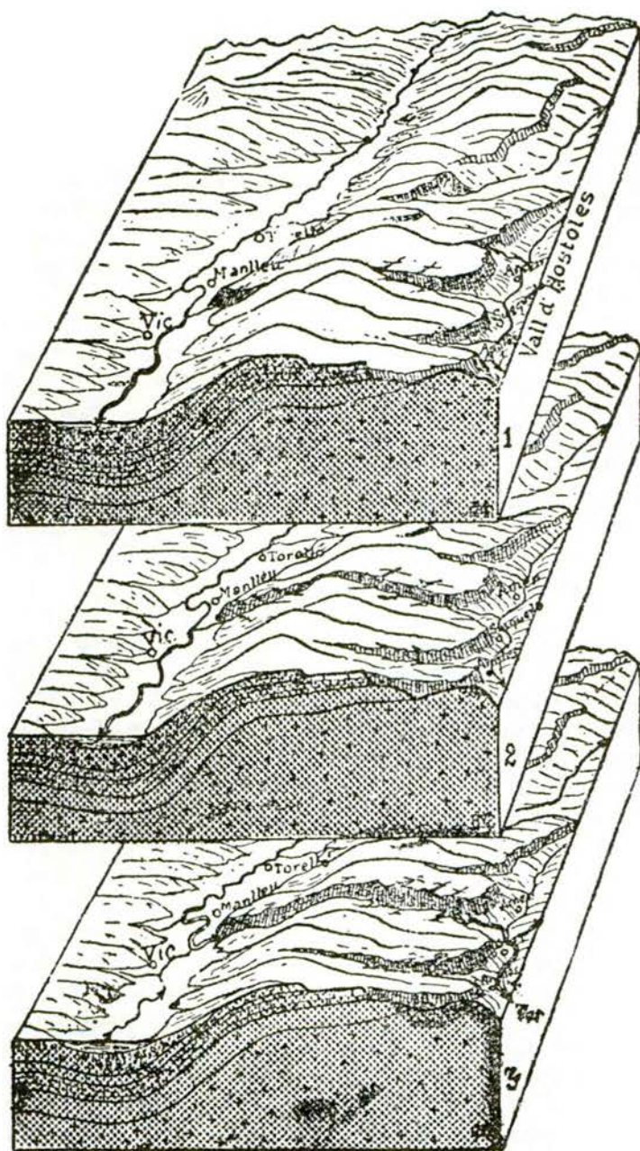
Fig. 9. - La desviació del Ter. segons M. Chevalier.
